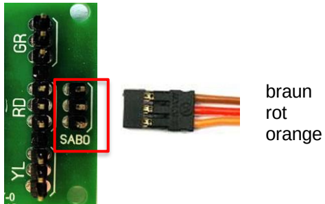
Abbildung 4: Steckeranschluss
